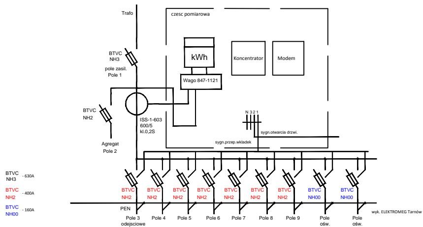
Schemat jednokreskowy rozdzielnic
