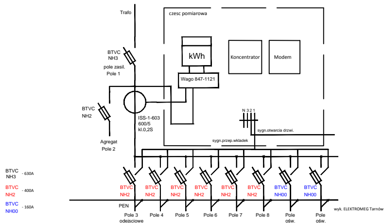
Schemat jednokresowy rozdzielnic
