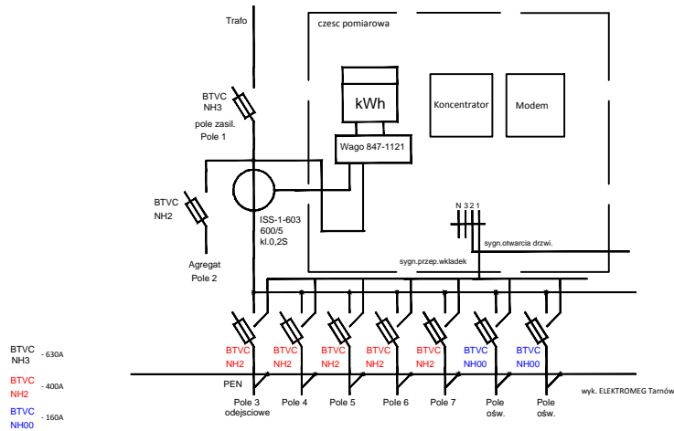
Schemat jednokreskowy rozdzielnic
