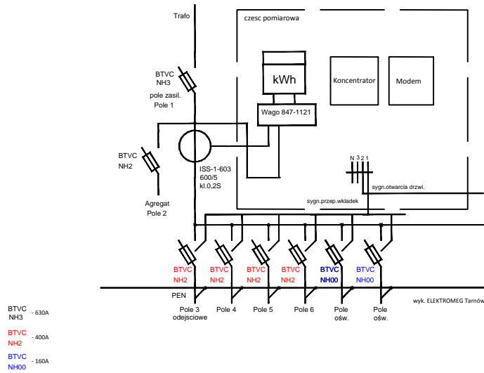
Schemat jednokreskowy rozdzielnic
