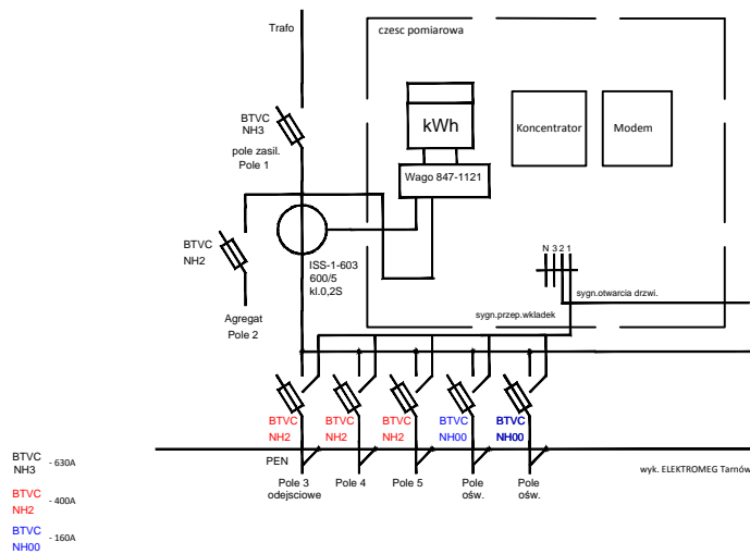
Schemat jednokreskowy rozdzielnic
